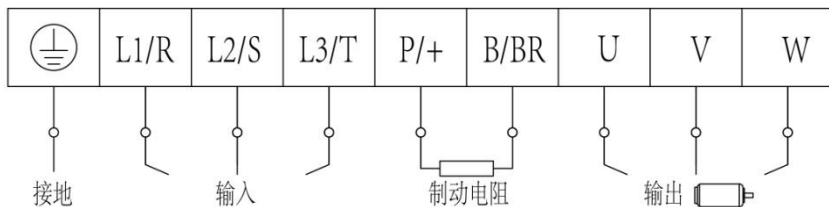
图 3-2 端子示意图
