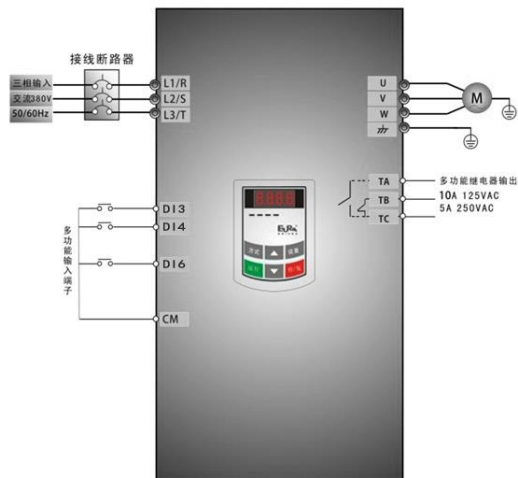
图 4-2 接线图 2
