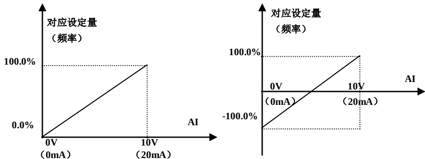
图 5-14 模拟给定与设定量的对应关系
