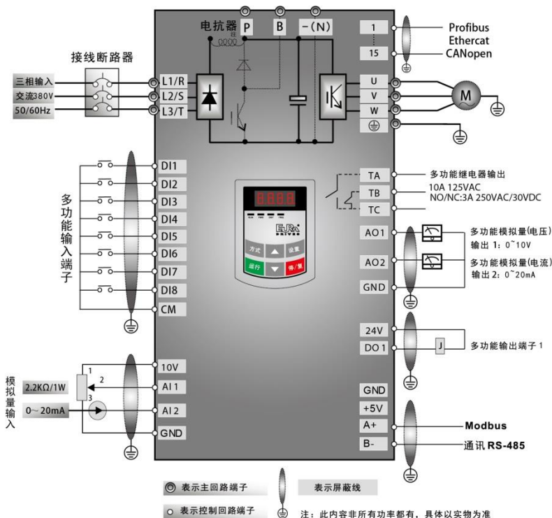
图 3-6 三相变频器标准配线图 (NPN 方式)
