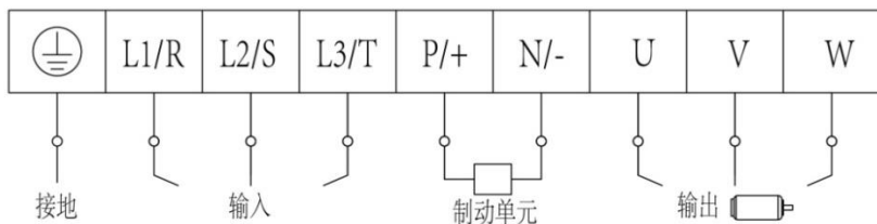
图 3-5 端子示意图
