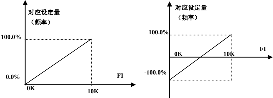
图 5-16 脉冲输入与设定量的对应关系
