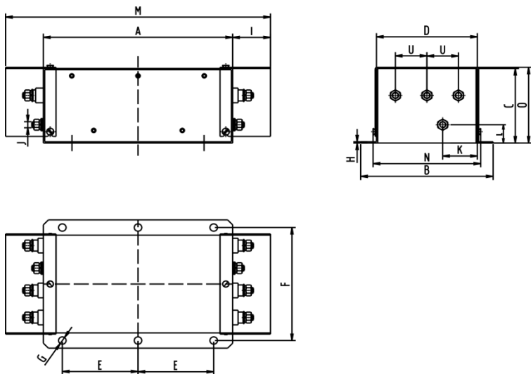
2、FN3359 外形尺寸及安装尺寸
