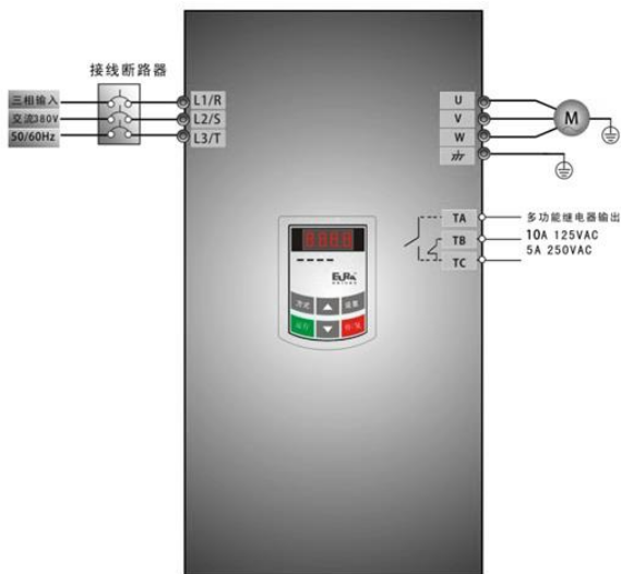
图 4—1 接线图 1
