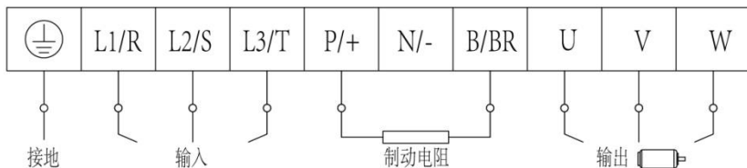
图 3-3 端子示意图
