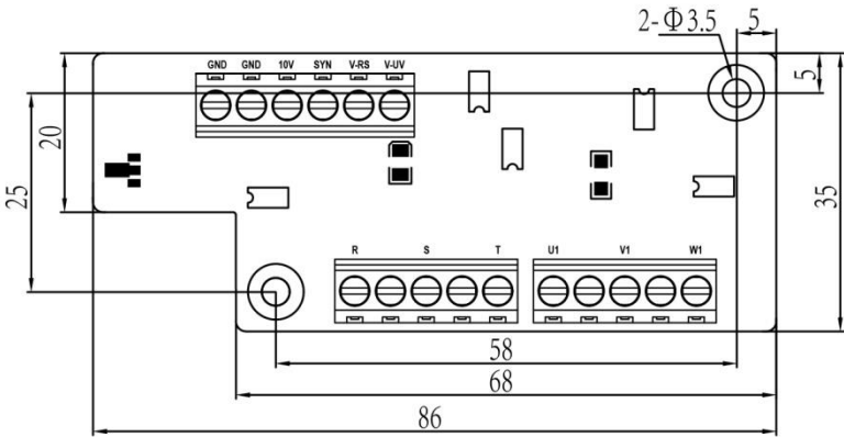
1. 1. 3、EPS 市电同步卡尺寸与安装说明如下图，单位（mm）
