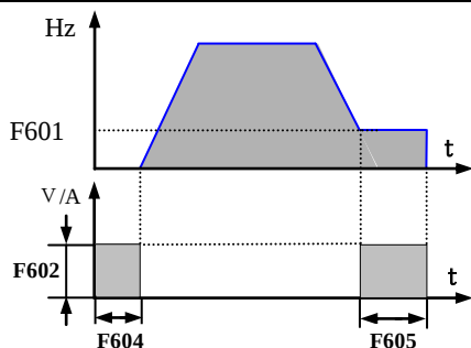
图 5-20 直流制动
