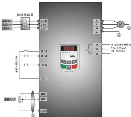
图 4-3 接线图 3
