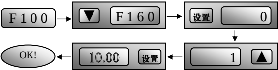
图 5-3 恢复出厂值
