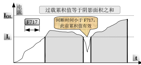
图 9-4 过载保护
