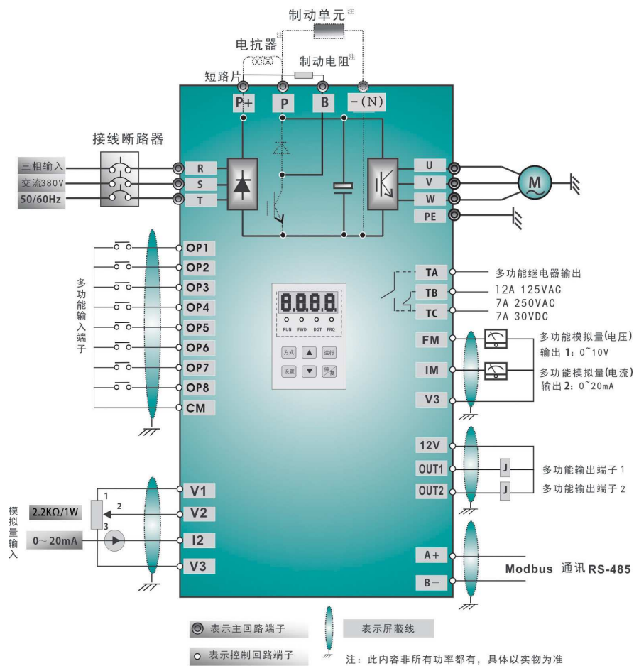
三相变频器标准配线图
