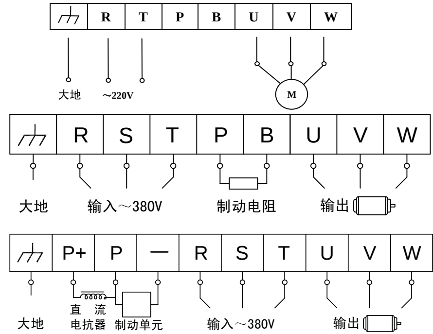
功率回路端子说明
