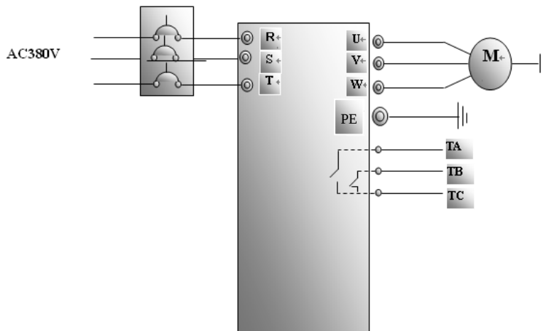
图 4-1 接线图 1
