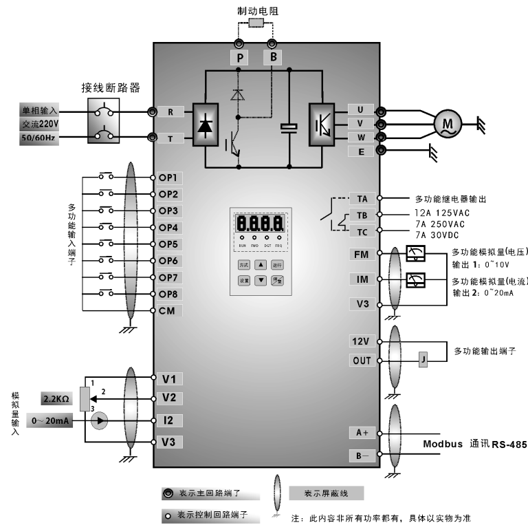
单相变频器标准配线图
