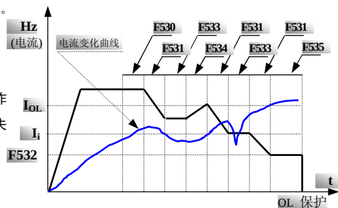
图 9-3 失速调节
