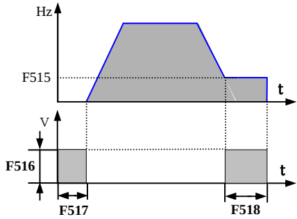
图 9-2 直流制动
