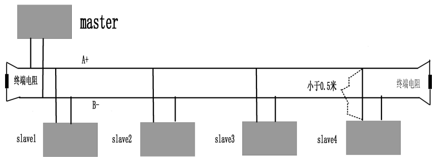
终端电阻连接图
